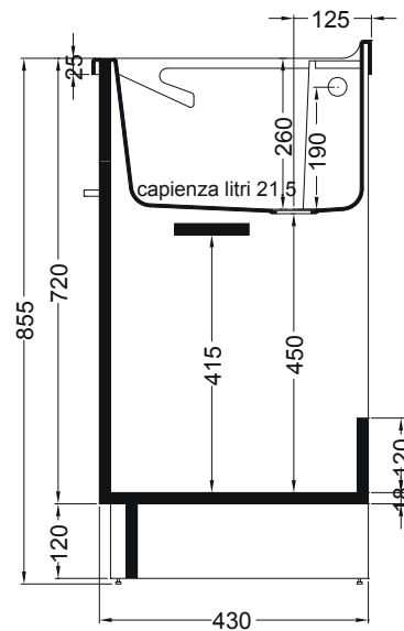
SEZIONE A-A'
