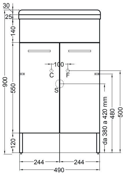
VISTA FRONTALE
