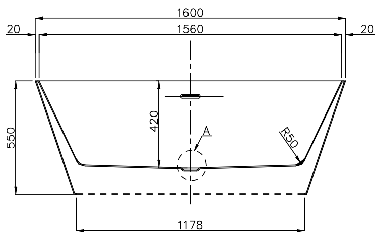
SEZIONE F-F
