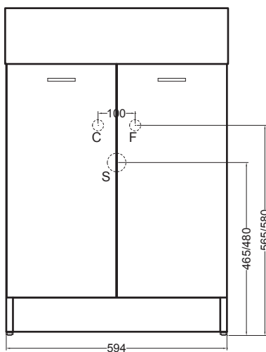
VISTA FRONTALE
